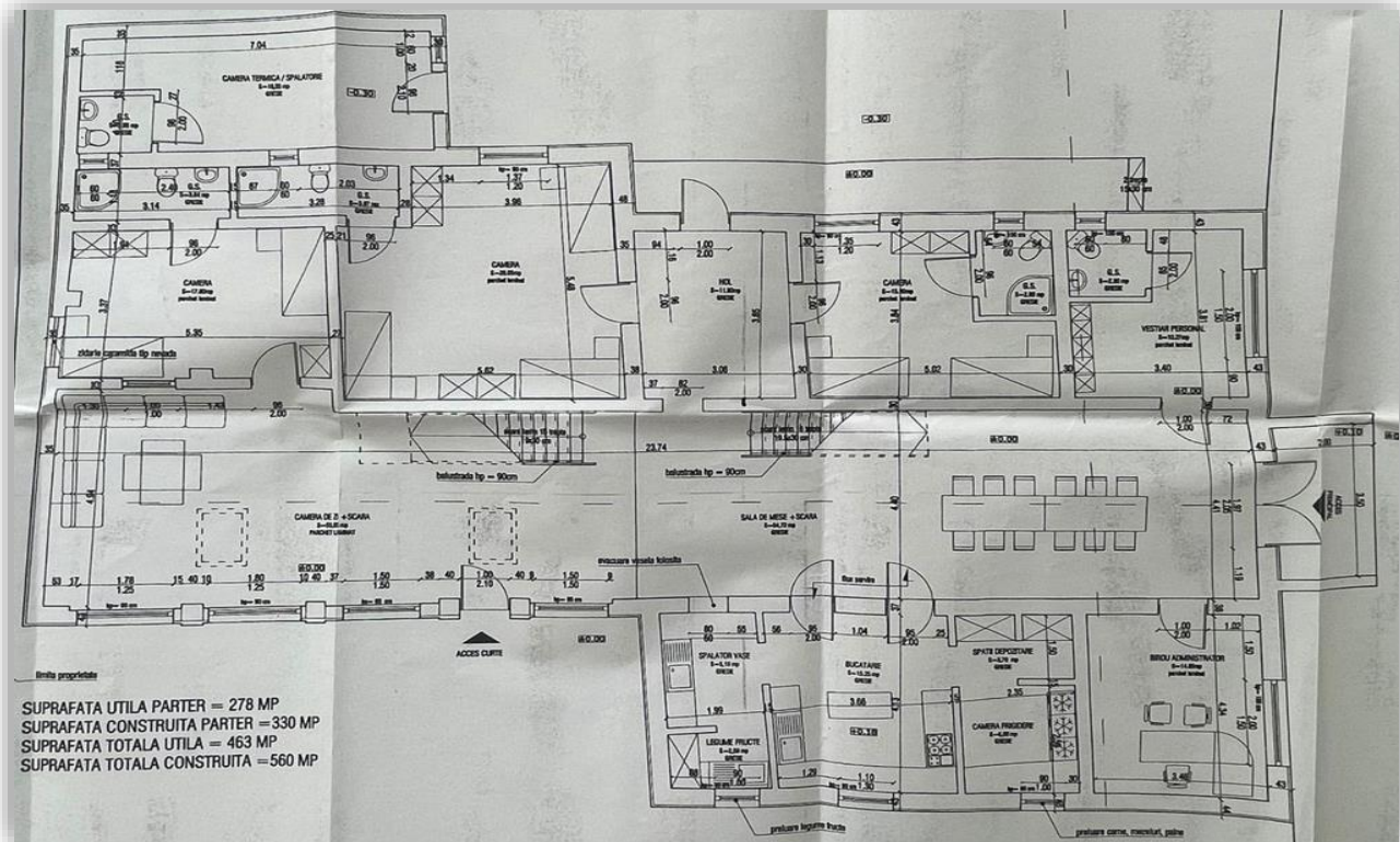
Fig.1 Grundriss des Erdgeschosses
